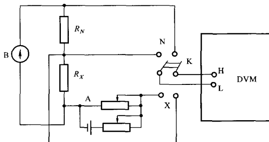
图 A1 数字电压表检定电阻箱的工作原理图
